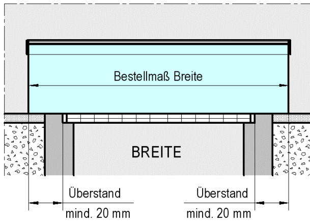
Schnittansicht Breite
