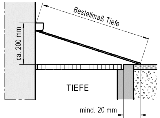
Schnittansicht Tiefe
